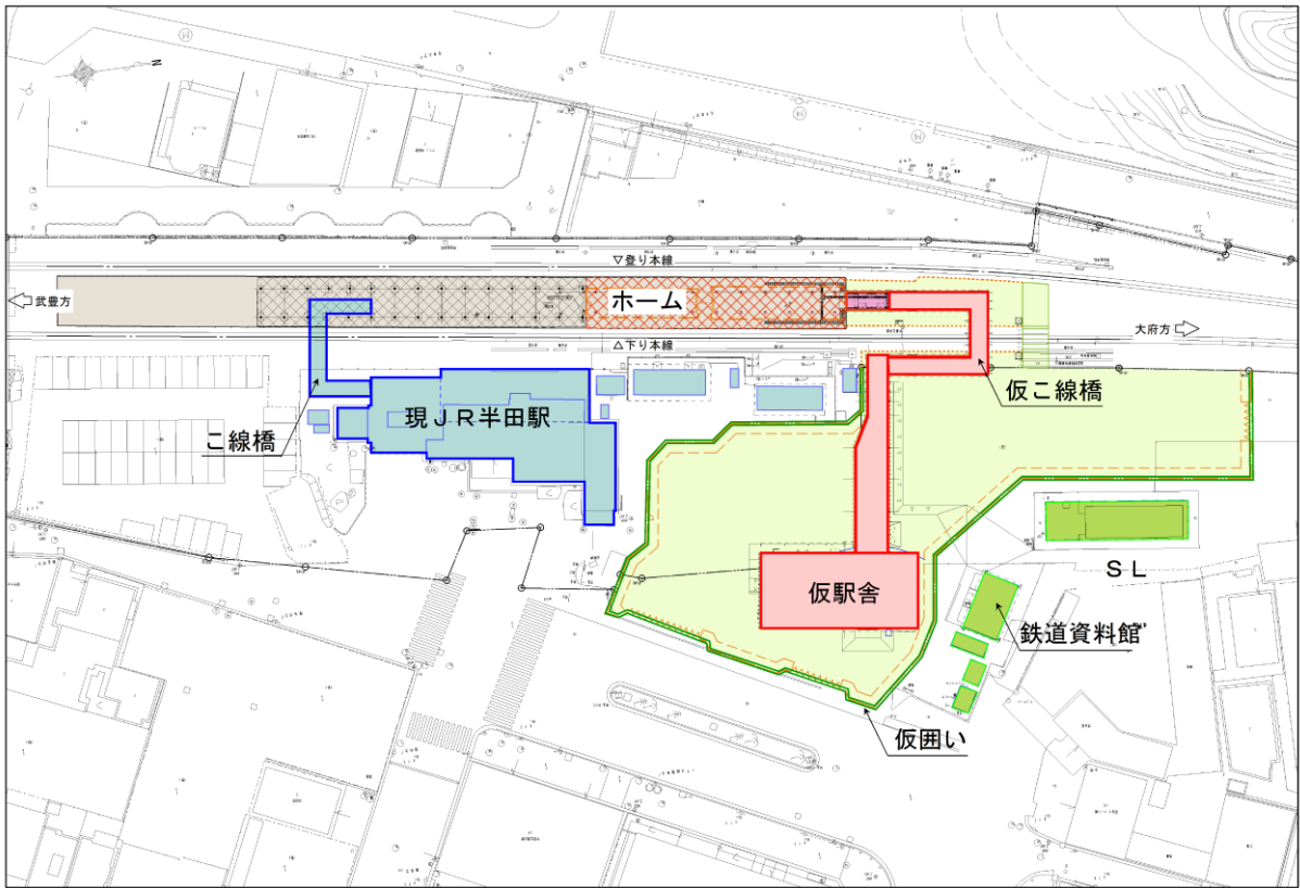
図面1 仮駅舎建設平面図
